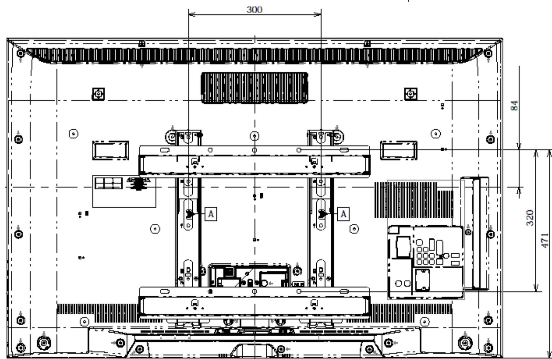
壁掛けユニット 取り付け時の寸法図
