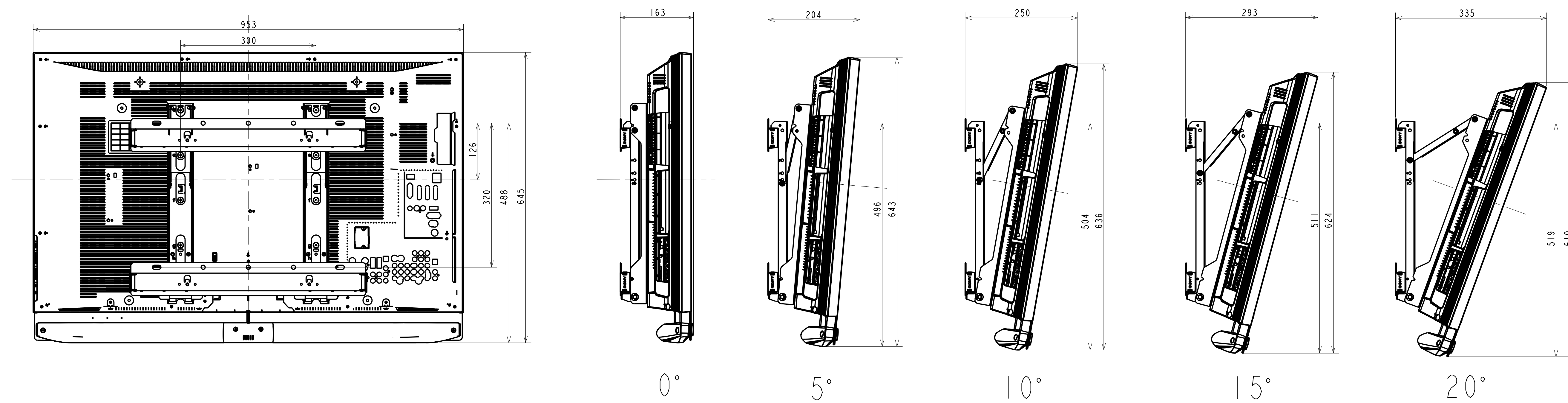
壁掛けユニット 取り付け時の寸法図
