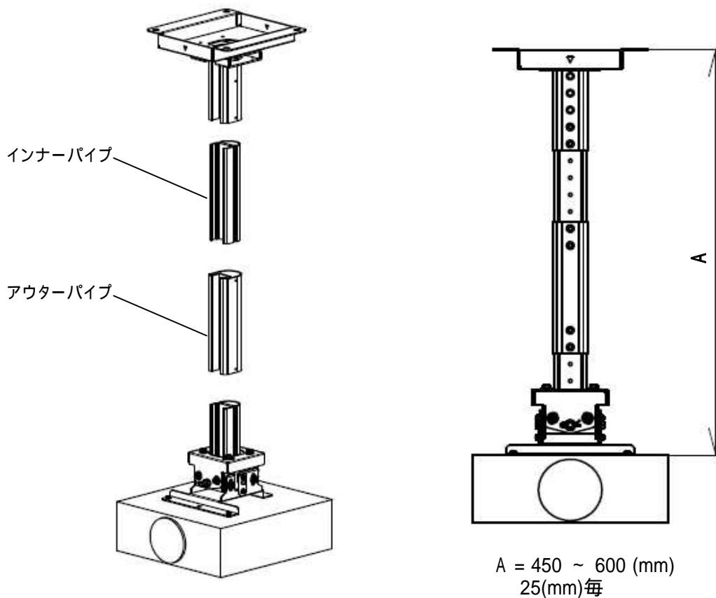
サスペンションサポートとの組合せによる組立状態図
