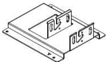
サスペンションサポートとの組合せによる組立状態図
